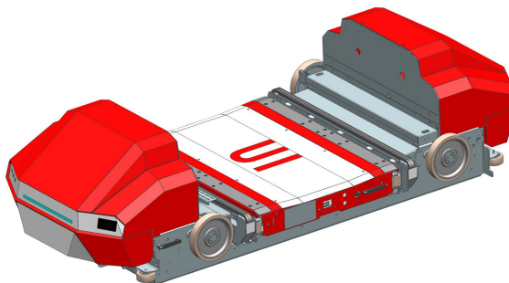
立体图
